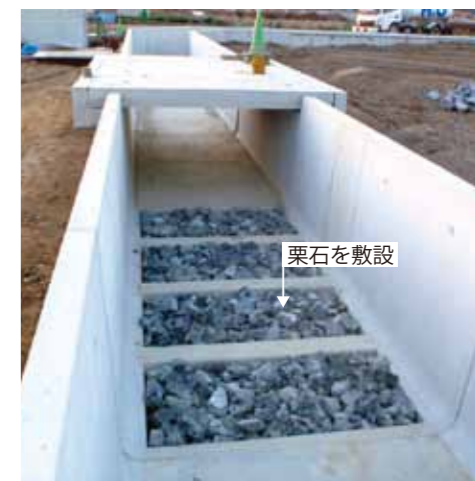
用水路 施工完了
